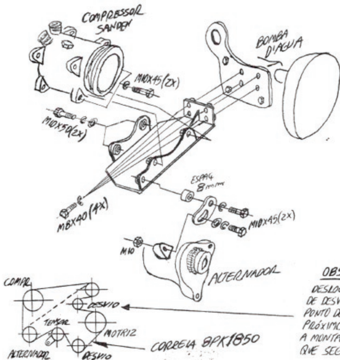
LAY-OUT DAS CORREIAS
